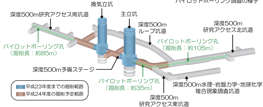
パイロットボーリング調査の様子
